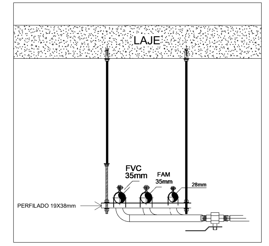
DETALHE SUPORTAÇÃO GASES
