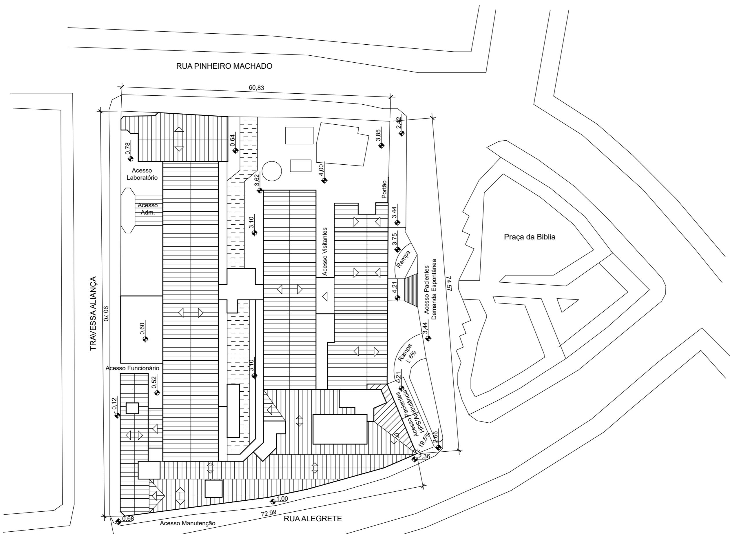
SITUAÇÃO ESCALA 1:500
