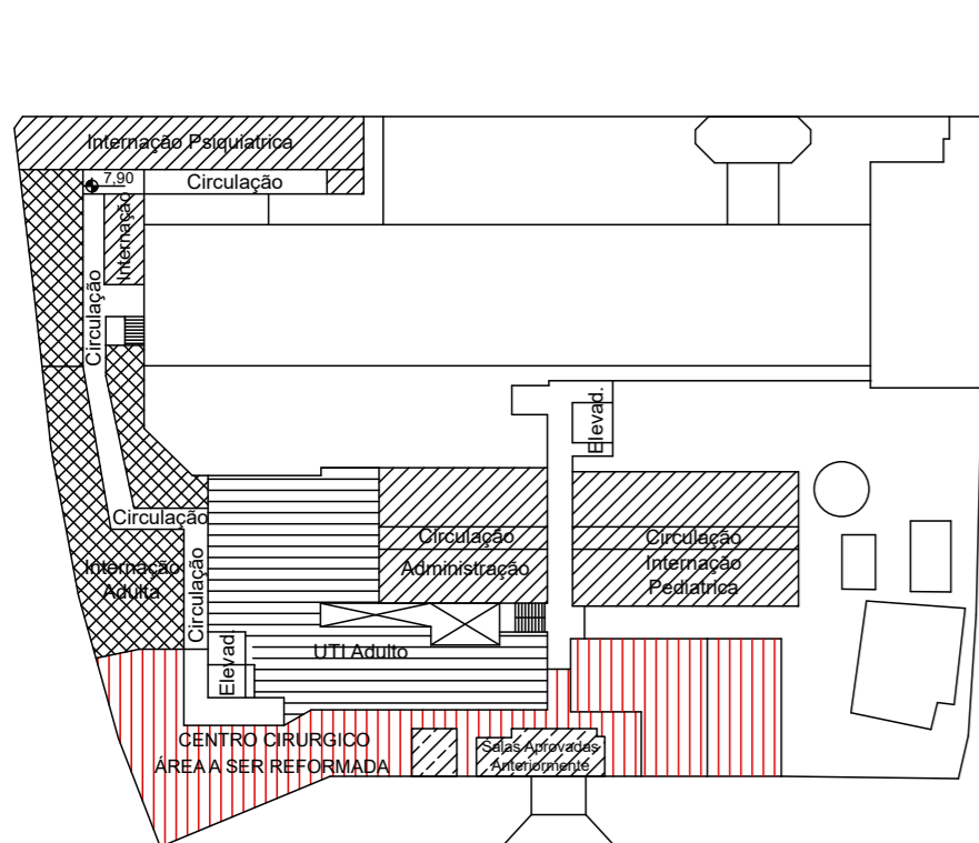
C.M.E. - 3º PAVIMENTO - Planta De Localização ESC. 1:750
