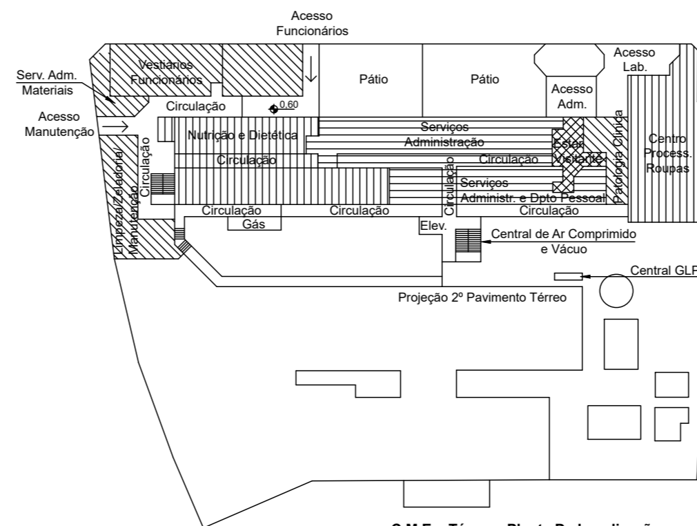
C.M.E. - Térreo - Planta De Localização ESC. 1:750
