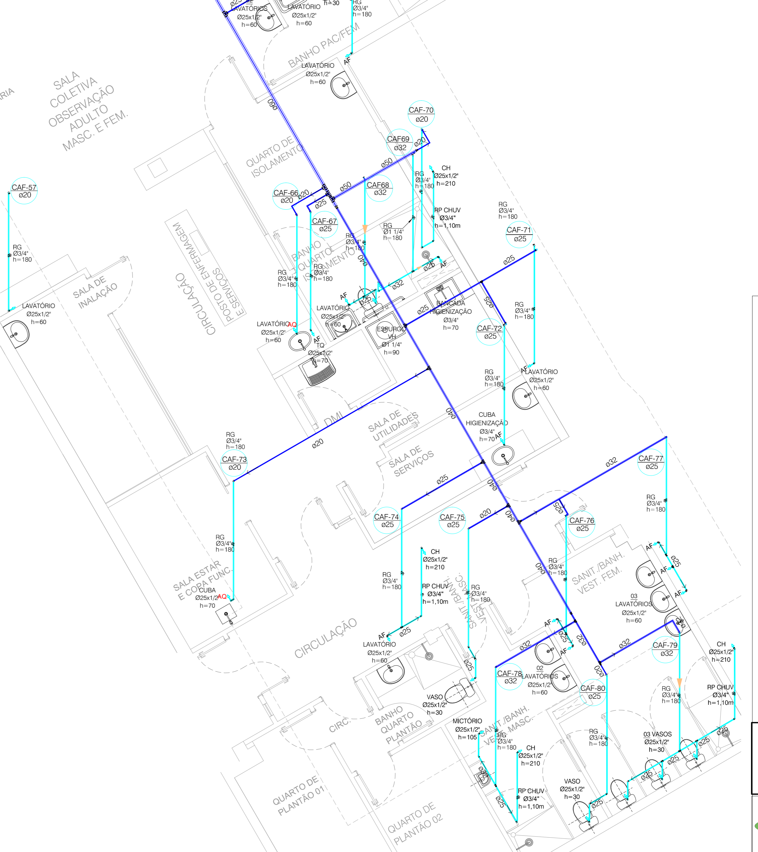
ESTEREOGRAMA PAVIMENTO TERREO - ÁGUA QUENTE E FRIA ESC:1/50
