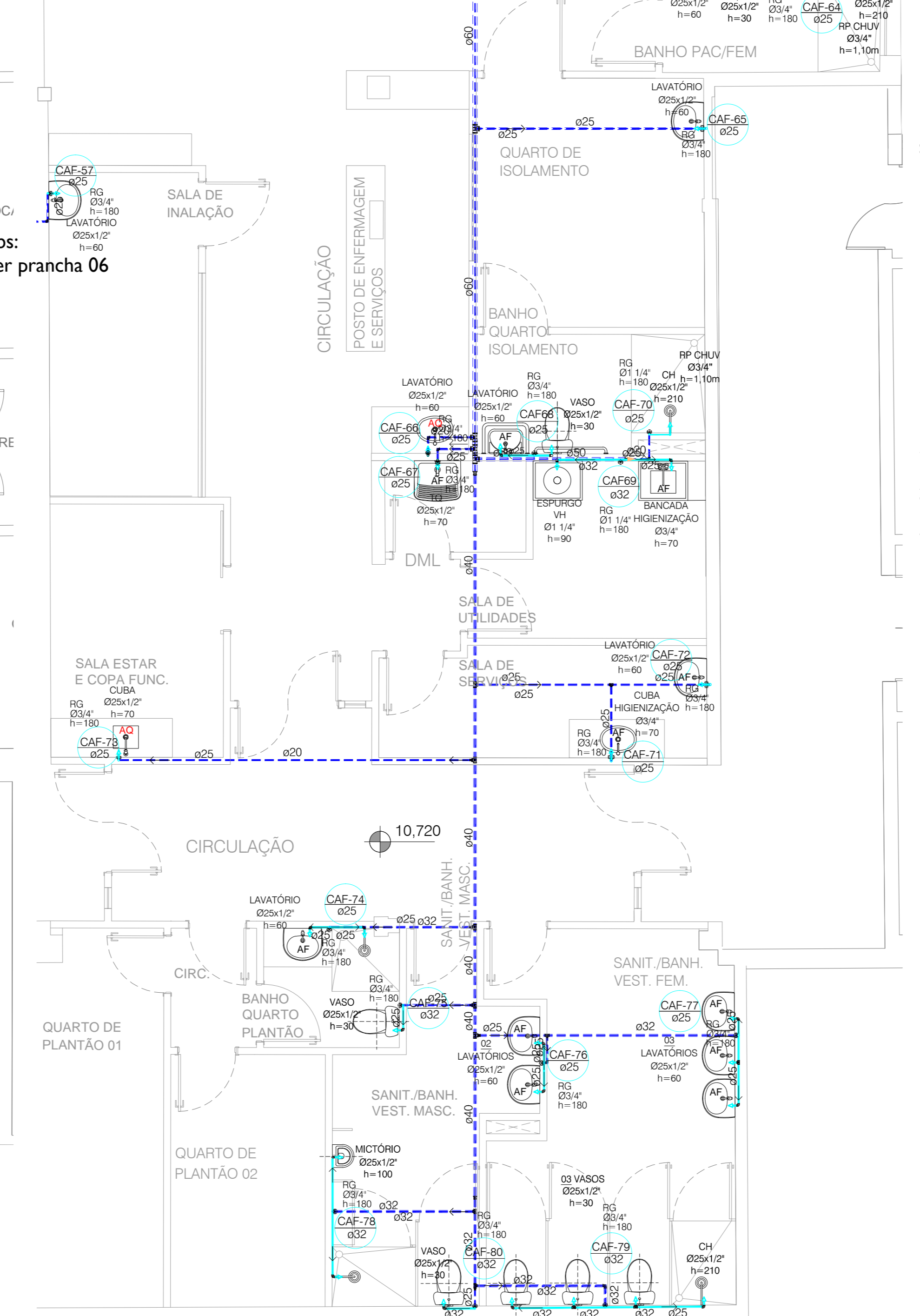
PLANTA BAIXA PAVIMENTO TERREO - ÁGUA QUENTE E FRIA ESC:1/50
