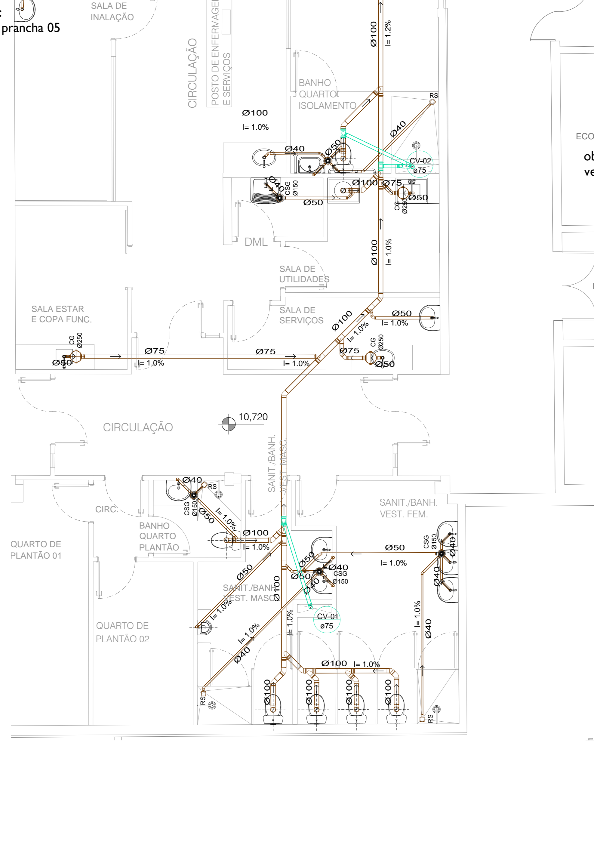
PLANTA BAIXA PAVIMENTO TERREO - ESGOTO ESC:1/50
