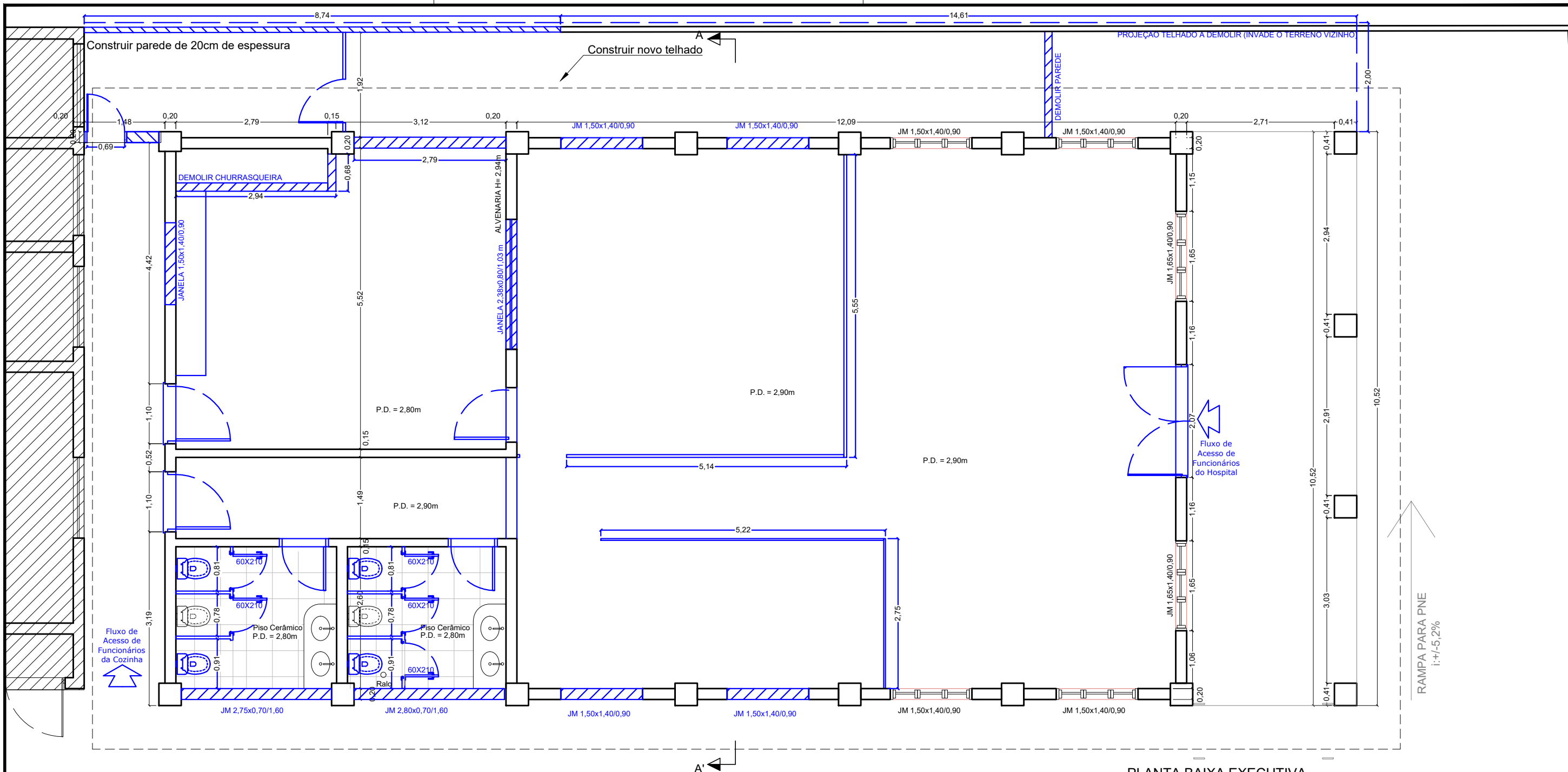
PLANTA BAIXA EXECUTIVA 1º PAVIMENTO - ESC. 1/75
