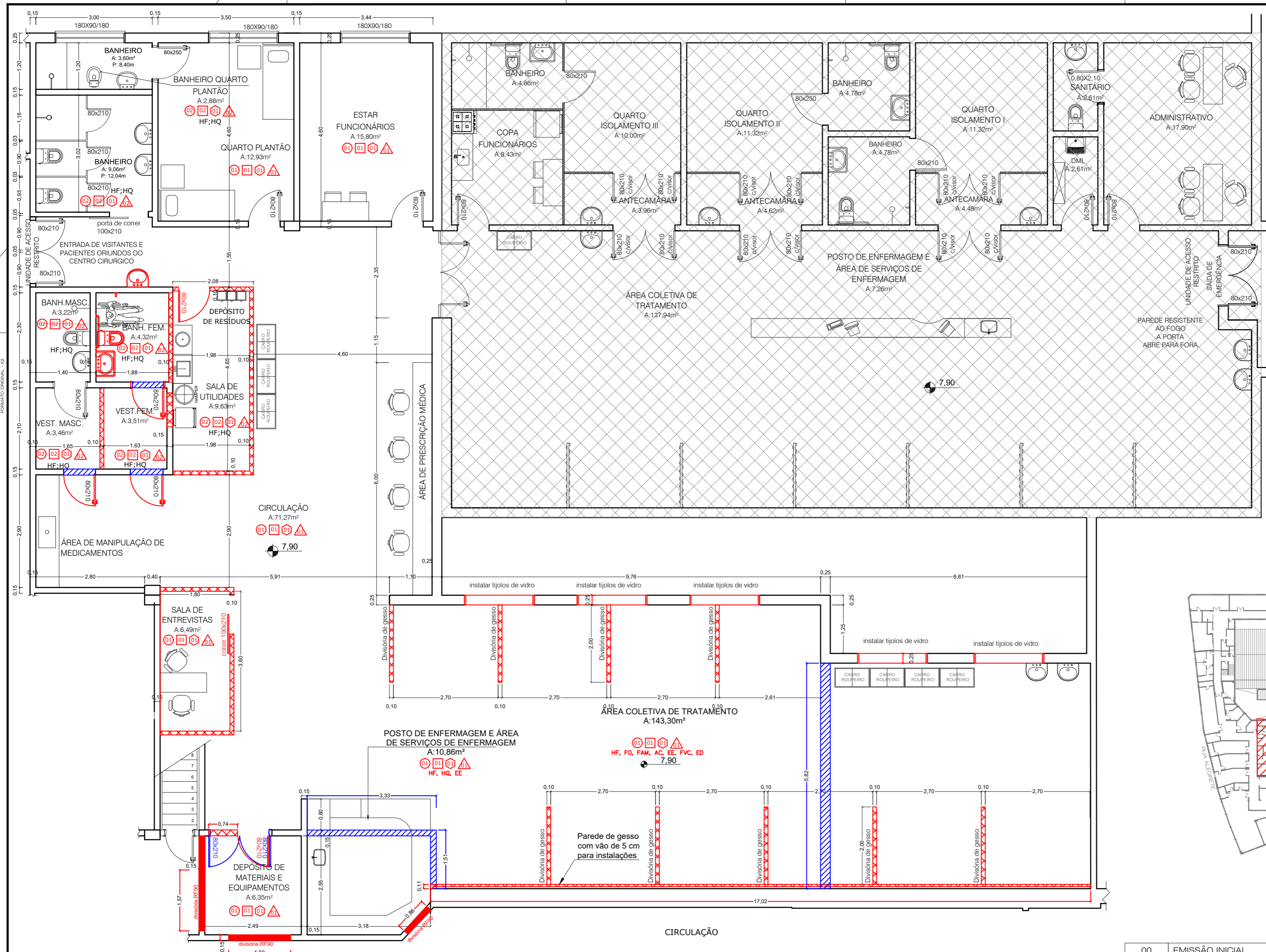
3º PAVIMENTO - Planta Baixa ESC. 1:75
